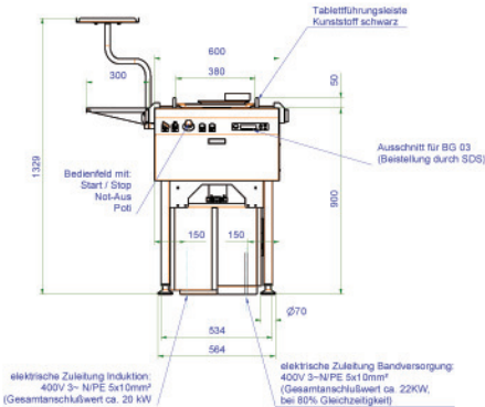
A (1 : 10)
