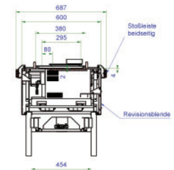
B-B (1 : 10)
